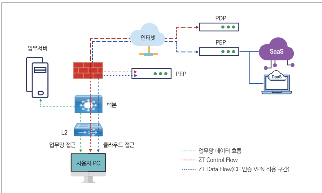
그림 S-2 클라우드 환경 제로트러스트 실증을 위한 실험망 구성도
