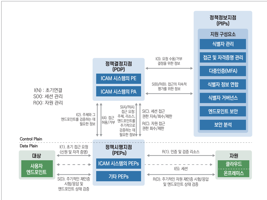
그림 S-12 EIG 초기 단계 참조 아키텍처
