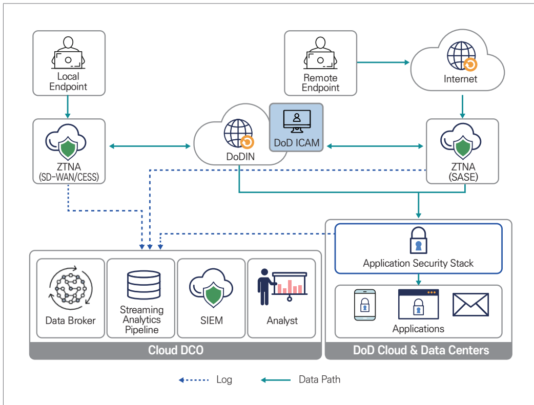
그림 S-13 Thunderdome 프로젝트 논리적 구성요소
