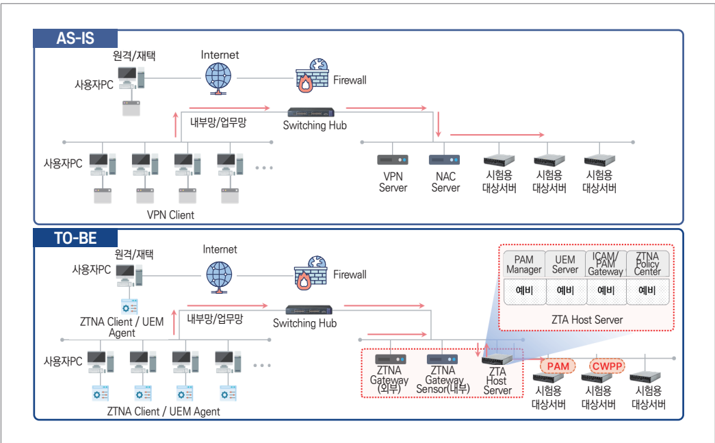
그림 S-8 온프레미스 통합 환경 제로트러스트 아키텍처 구성 도입 이후 개선 시스템 비교
