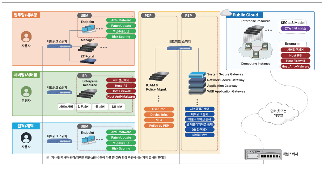
그림 S-7 온프레미스 통합 환경 제로트러스트 아키텍처 물리적 구성도
