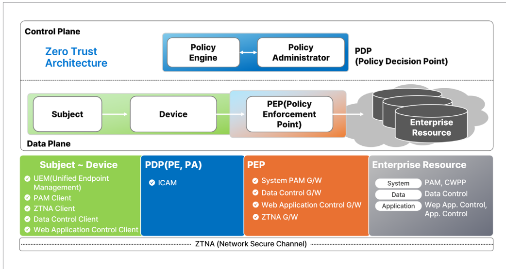
그림 S-5 온프레미스 통합 환경 제로트러스트 실증을 위한 환경 구성
