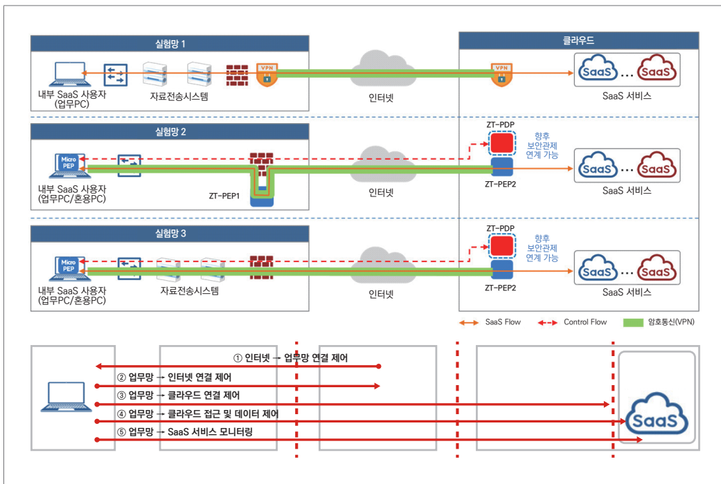
그림 S-3 클라우드 환경 제로트러스트 실증 시나리오 개념도
